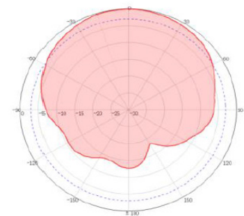
E-Plane
